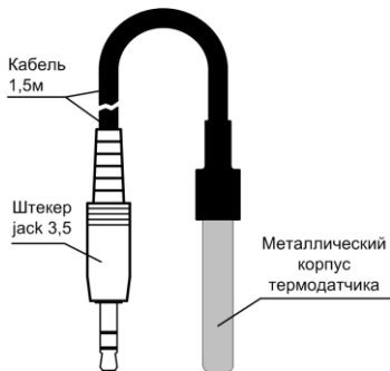
Рис.3 Внешний термодатчик
